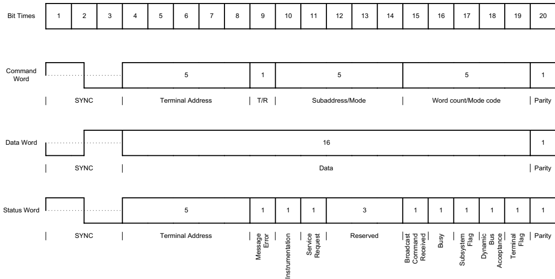
Fig. 4. Messages formats
