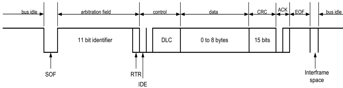
Fig. 2. CAN message format
