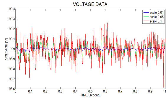
Fig. 3 Voltage data
