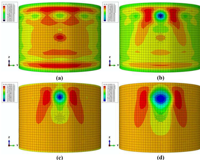
Fig. 5 Buckling mode shape corresponding to peak load: (a) 100%; (b) 92%; (c) 57%; (d) 36%
