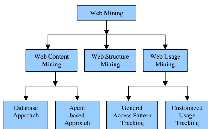
Fig. 2 Web Classification
