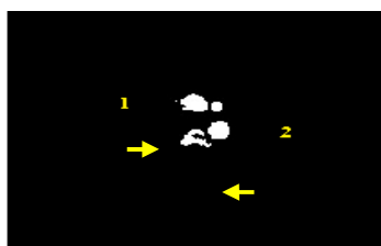
Fig. 4 1- AscA 2- DesA
