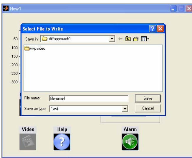
Fig. 8 GUI-5
