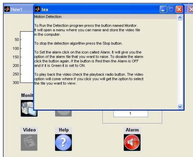
Fig. 5 GUI-2
