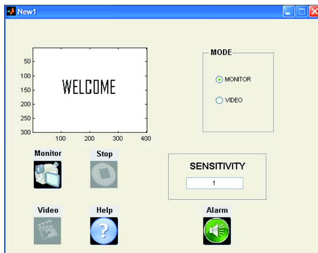
Fig. 10 GUI-7
