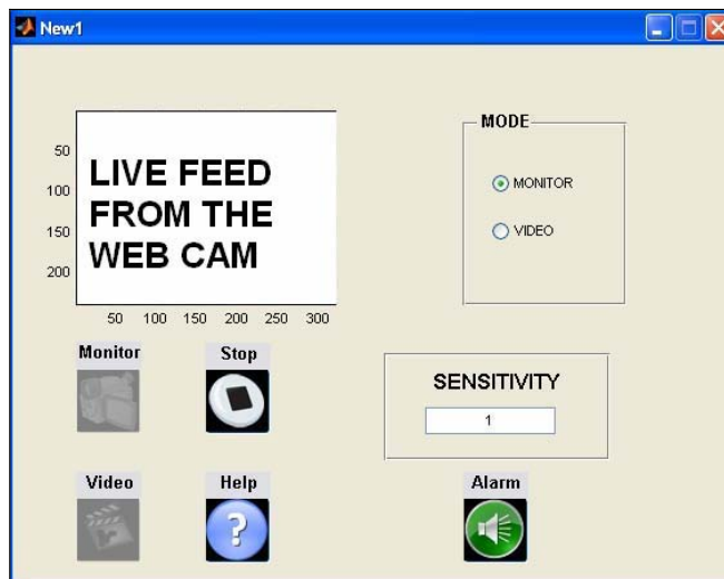
Fig. 9 GUI-6
