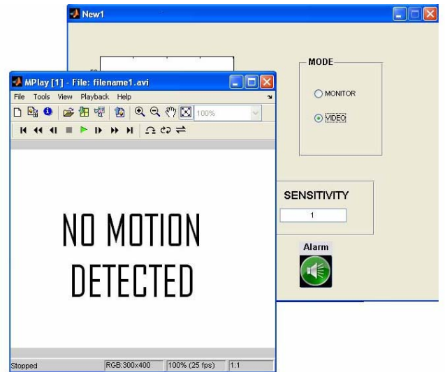
Fig. 14 GUI-11
