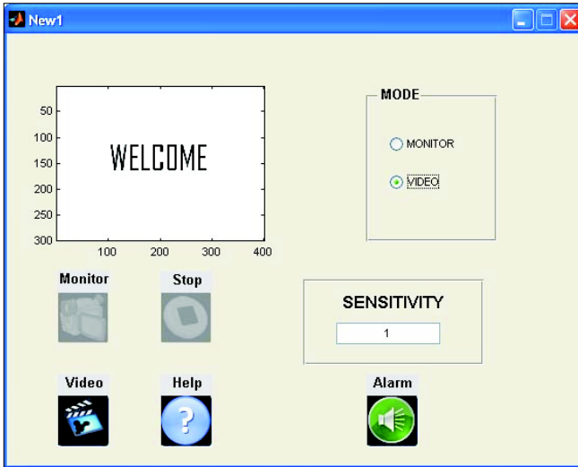
Fig. 11 GUI-8
