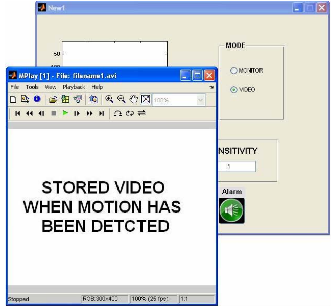
Fig. 13 GUI-10
