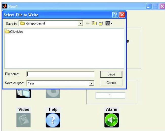
Fig. 7 GUI-4
