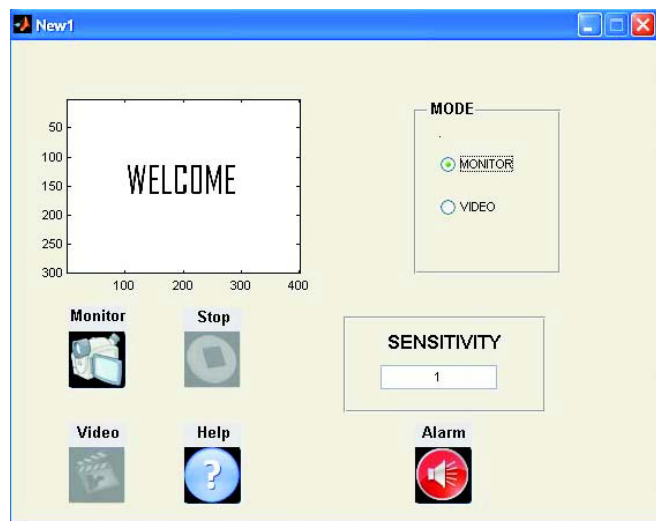
Fig. 4 GUI-1
