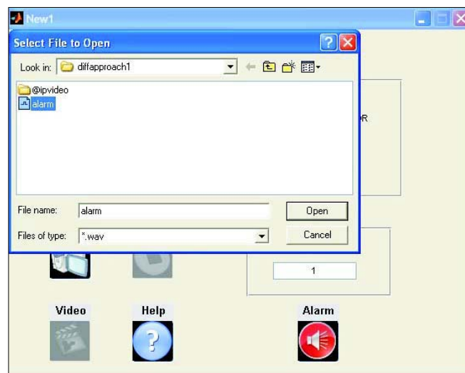
Fig. 6 GUI-3
