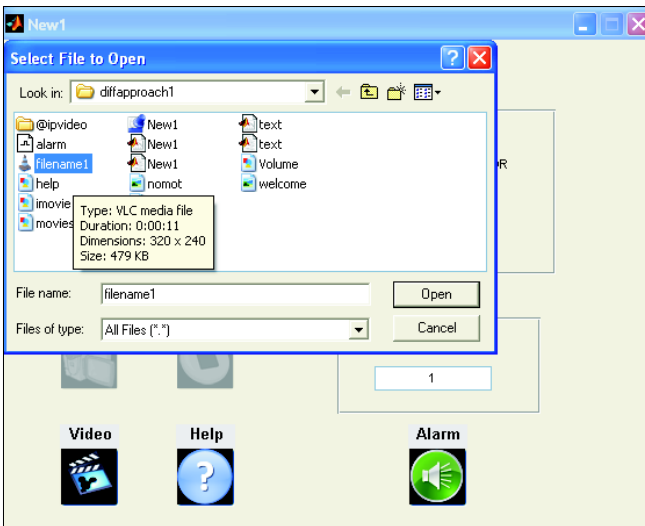
Fig. 12 GUI-9
