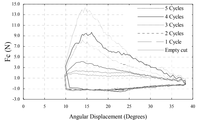
Fig. 8 Force-displacement data
