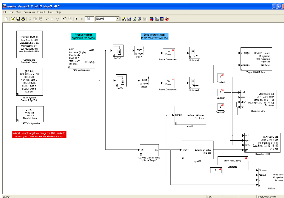
Fig. 7 Simulink model
