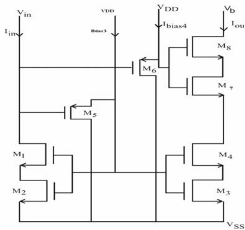
Fig. 4 Self Cascode LVCM
