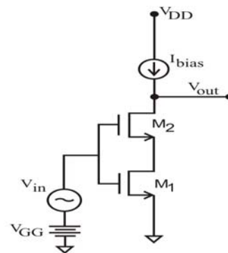
Fig. 3 Composite Cascode
