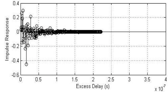
(b) NLOS
