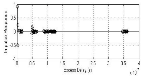
(a) LOS
