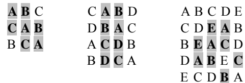
a. 4 pairs, K = 4/9 b. 4 pairs, K = 4/16 c. 5 pairs K = 5/25
