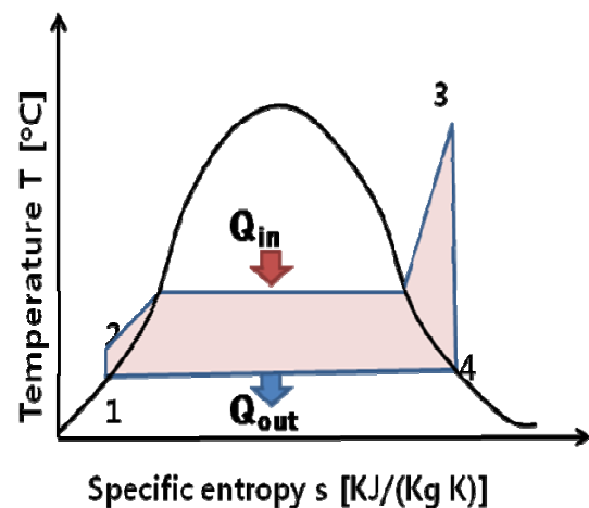
Fig. 2 T-s diagram
