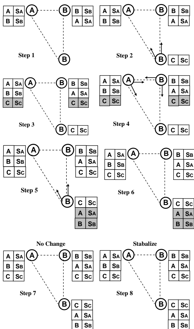
Fig 6: Scenario: Step 1 – 8
