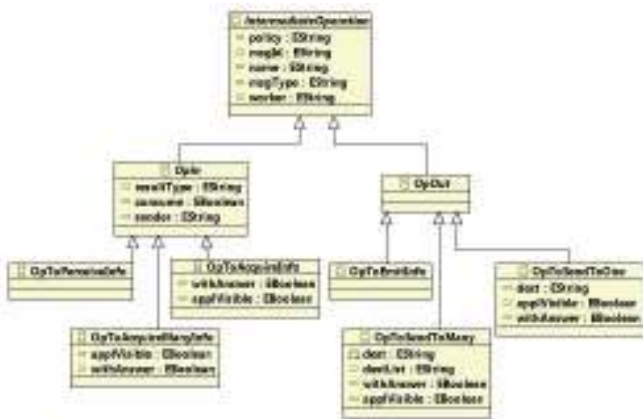
Fig. 4. The medcl meta-model
