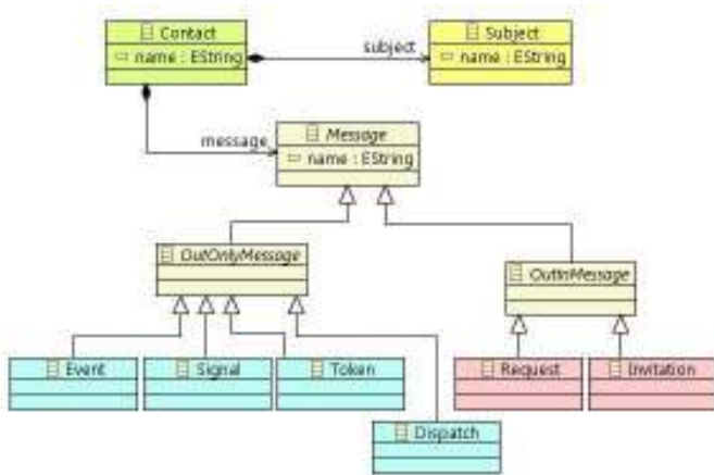
Fig. 1. Message ontology.
