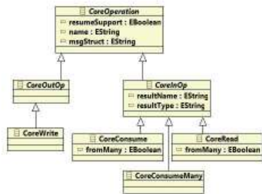
Fig. 5. The corecl meta-model
