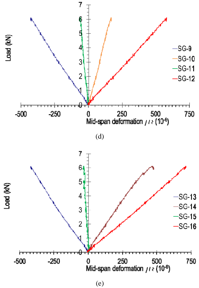
Fig. 4 Mid-span deflection (a), deformation (b) B-1, (c) B-2, (d) B-3 and (e) B-4
