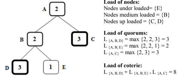
Fig. 6 Example load
