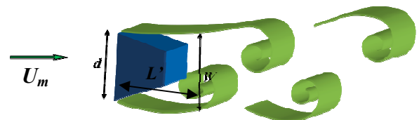
Fig. 2 Flow Parameters [5]
