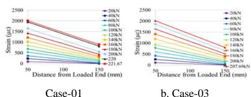
Case-01 b. Case-03 Fig. 18 Strain Profile of SA Specimens
