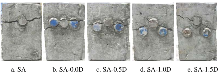
Fig. 15 Fracture Pattern of SA
