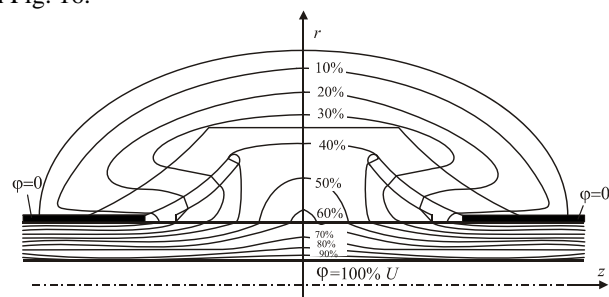
Fig. 16 Equipotential lines
