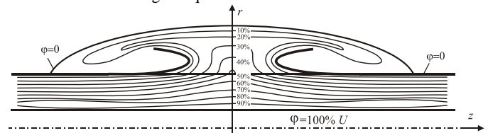
Fig. 5 Axial cross-section of equipotential surfaces
