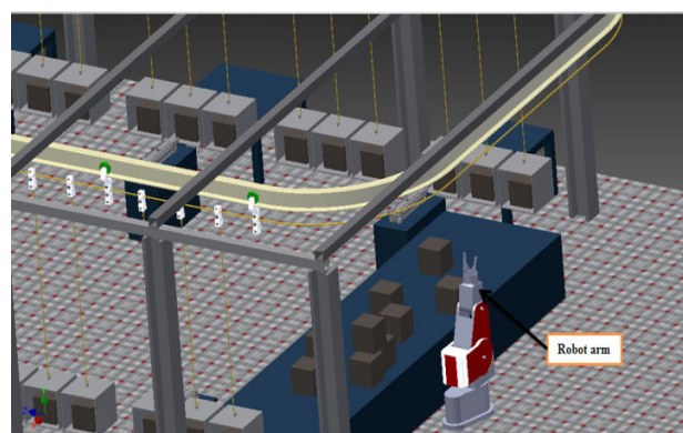
Fig. 2 Robot arm
