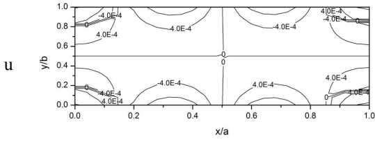
(d) \Omega/\omega_1=3.8237
