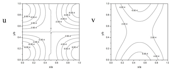
(d) \Omega/\omega_1 = 1.8677
