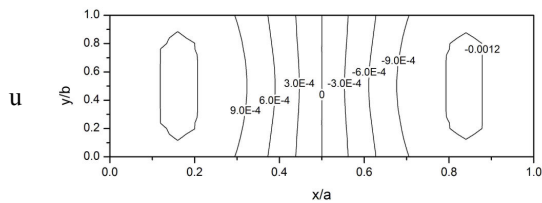
(d) \Omega/\omega_1=3.8237
