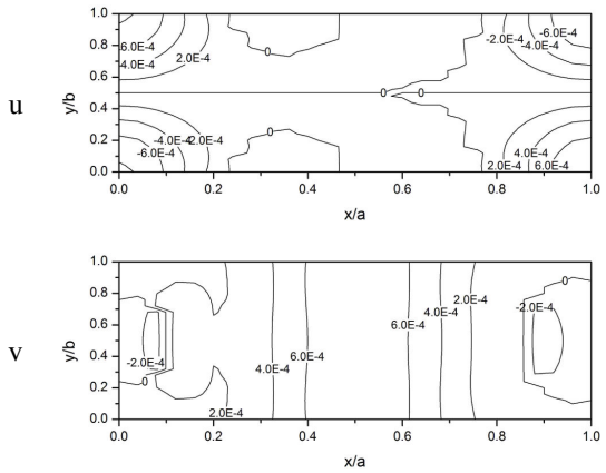
(d) \Omega/\omega_1 = 3.7813
