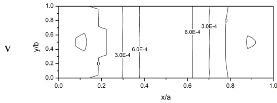
(d) \Omega/\omega_1=3.8237
