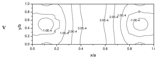
(d) \Omega/\omega_1=3.8237
