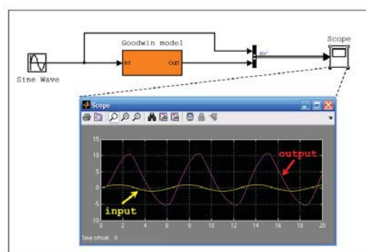
Fig. 22. Simulation of sinusoidal input
