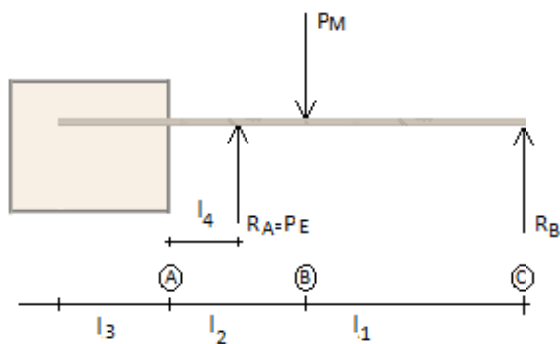
Fig. 5 Test Setup
