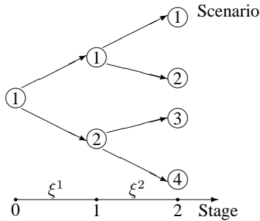
Fig. 1. Scenario tree
