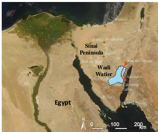
Fig. 1 Study area location (Wadi Watier)
