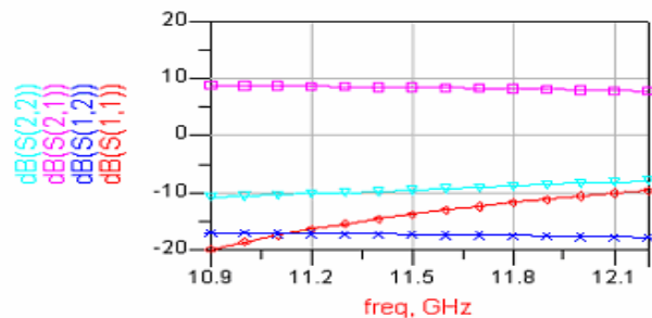
Fig. 10 S Parameters
