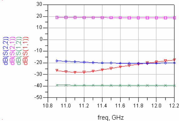
Fig. 16 S parameters
