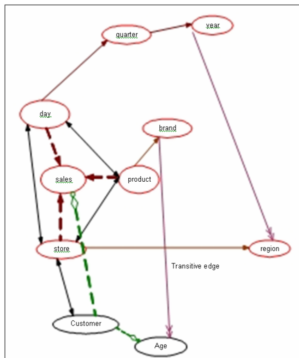
Fig. 3 A Data warehouse Schema
