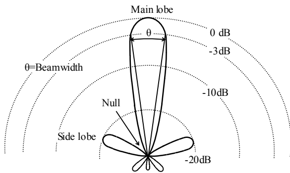
Fig. 1 Beamwidth
