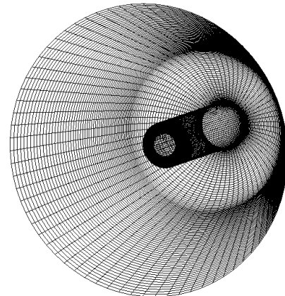
Fig. 3 Nose-tip surface grid ( L=32\text{mm} , D=8\text{mm} )
