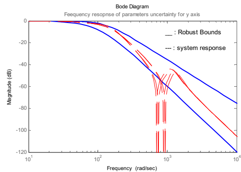
(d) Frequency responses of Y axis
