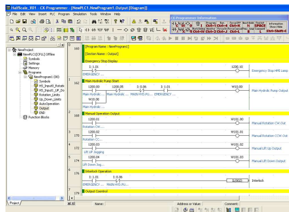
Fig. 9 CX-Programmer
