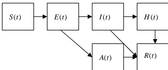
Fig. 3 SEIAHR model
