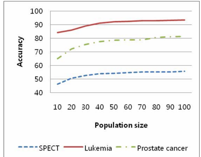
Fig. 2 Accuracy per population size
