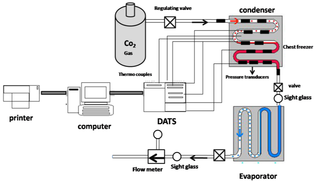
Fig. 1 Tests Apparatus
