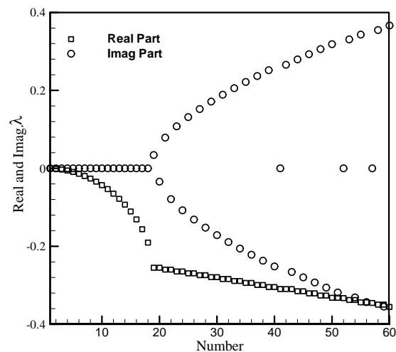
Fig. 7 The first 60 eigenvalues in \lambda -plane
