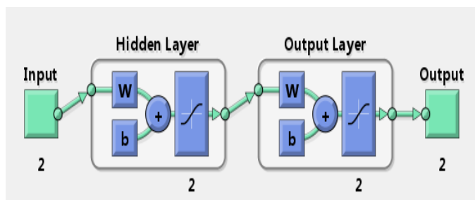
Fig. 8 ANN structure
