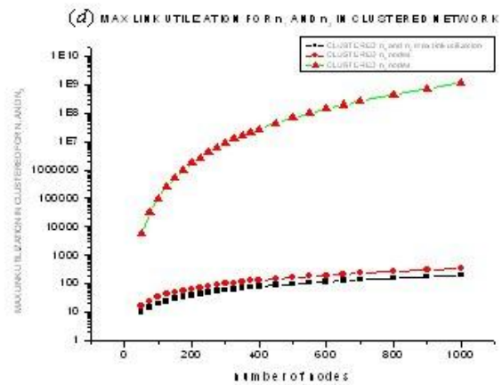
Fig. 7. Maximum Link Utilization (c) and (d) (upper bound)
