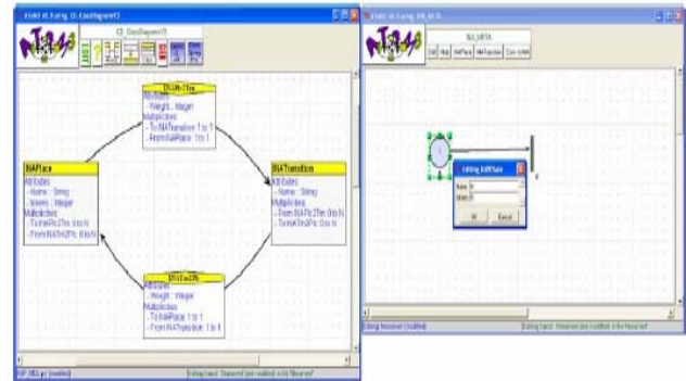
Fig. 4 (a) INA PN Model (b) INA Tool
