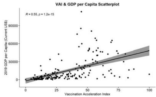
Fig. 7 Scatterplot of VAI and GDP per capita
