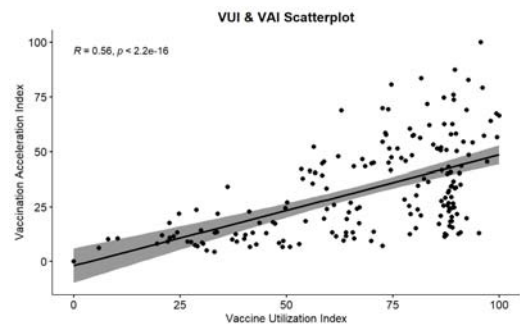
Fig. 3 Scatterplot of VUI and VAI
