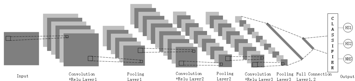
Fig. 1 CNN
