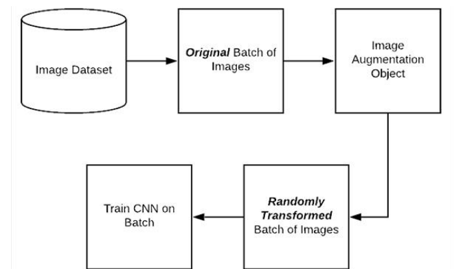
Fig. 3 Data Augmentation
