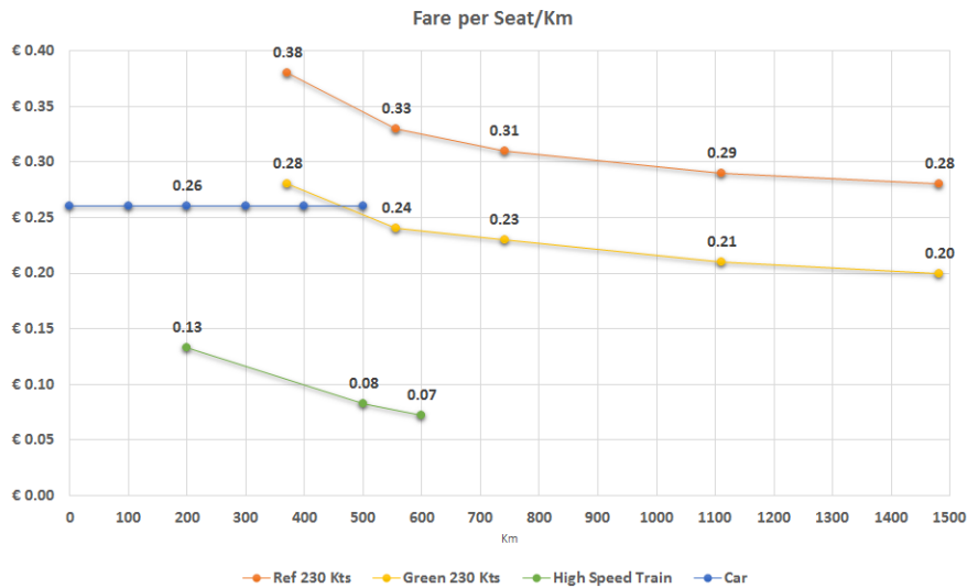
Fig. 20 Fare per seat/km
