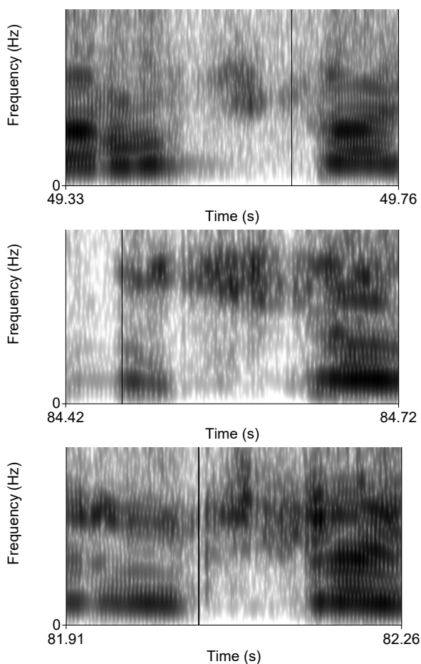
Fig. 7 Contour spectrogram of the word «ručka»
