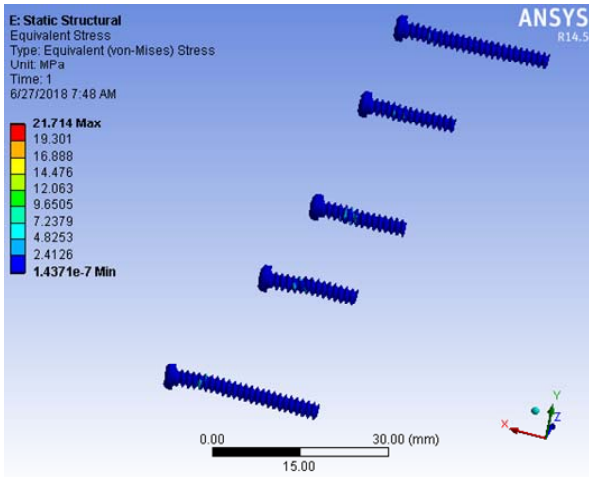
Fig. 5 (d) Von-Mises stress distribution in all screws
