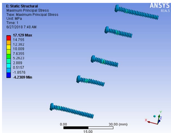
Fig. 6 (d) Maximum principal stress in all screws
