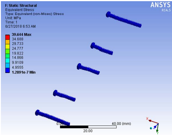
Fig. 5 (d) Von-Mises stress distribution in all screws
