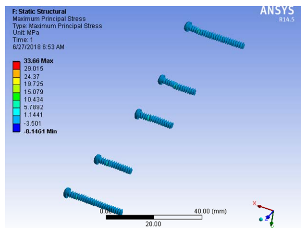
Fig. 6 (d) Maximum principal stress in all screws
