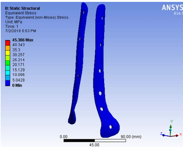
Fig. 7 (d) Von-Mises stress distribution in implants
