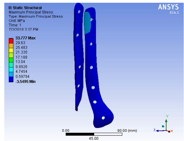
Fig. 8 (d) Maximum principal stress in implants
