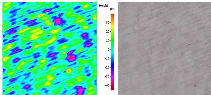
Fig. 4 Sandblasting
