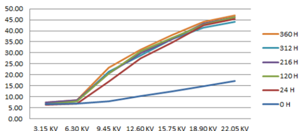
Fig. 8 Tan delta trend of AS01 (VPI system)
