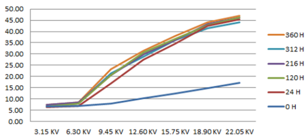
Fig. 8 Tan delta trend of AS01 (VPI system)
