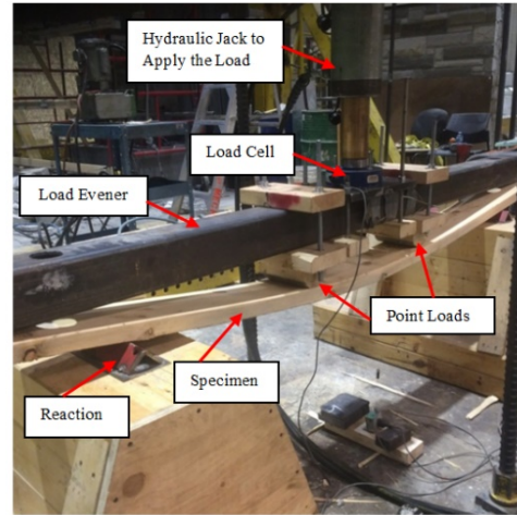
Fig. 3 Stud bending test setup
